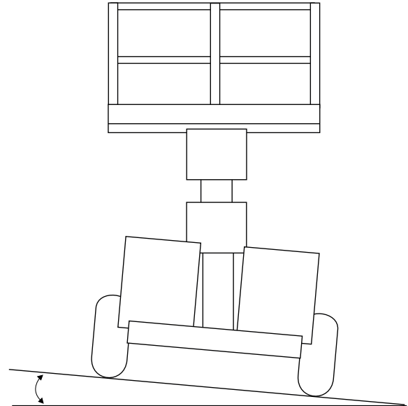
13° Seite/Seite
